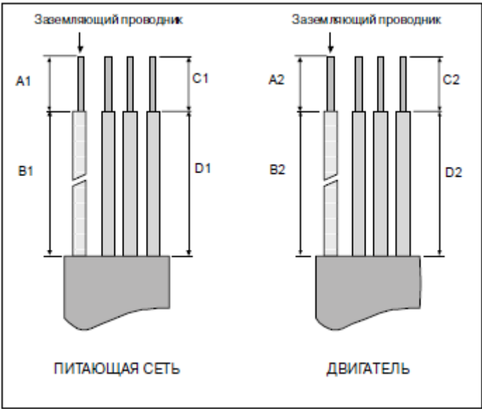
Рисунок 5-2. Зачистка кабеля
