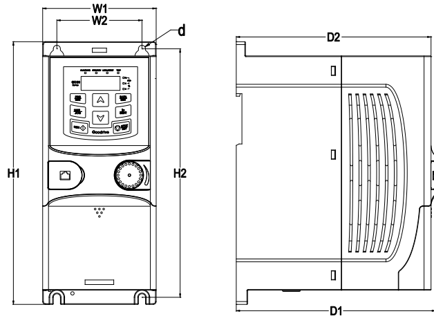
Рис. 4.6 Настенный монтаж 0.4 – 2,2 кВт
