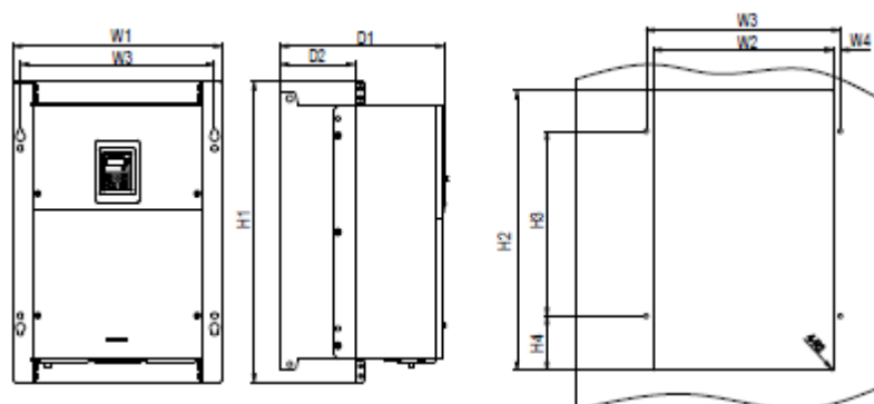
Рис. 4.12 Фланцевый монтаж 90 – 110 кВт
