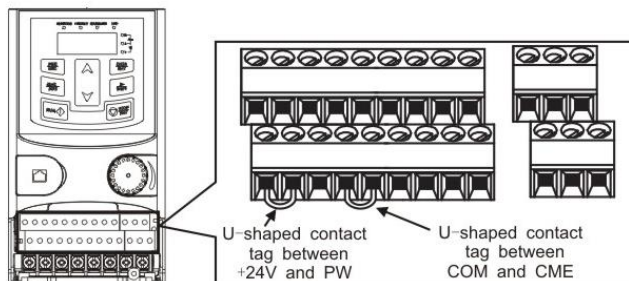
Рис.5-18 U-образный контакт
