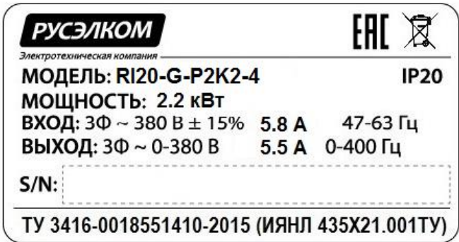
Рисунок 2-1. Шильдик преобразователей частоты RI20
