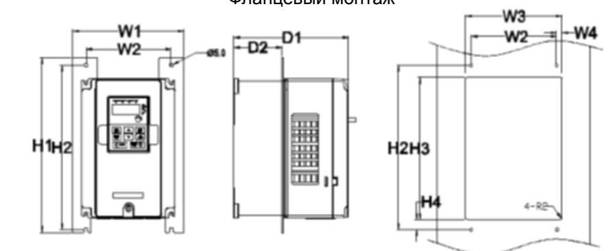
Рис. 4.11 Фланцевый монтаж 4 – 75 кВт
