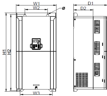
Рис. 4.9 Настенный монтаж 45 – 75 кВт
