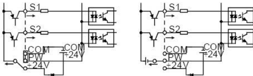
Рис.5-20 PNP режим
