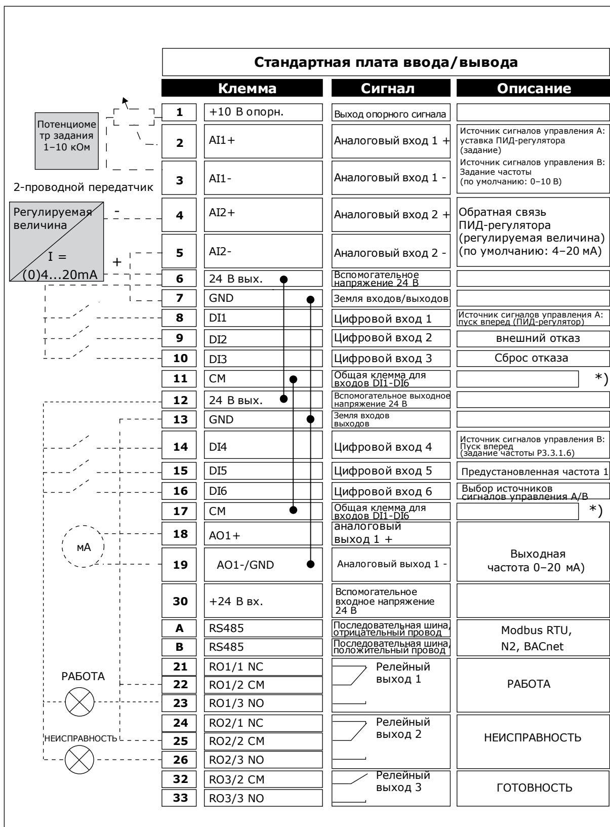
Рис. 10: Цепи управления, которые по умолчанию используются для приложения ПИД-регулятора
