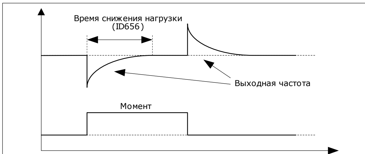
Рис. 21: Функция снижения нагрузки
