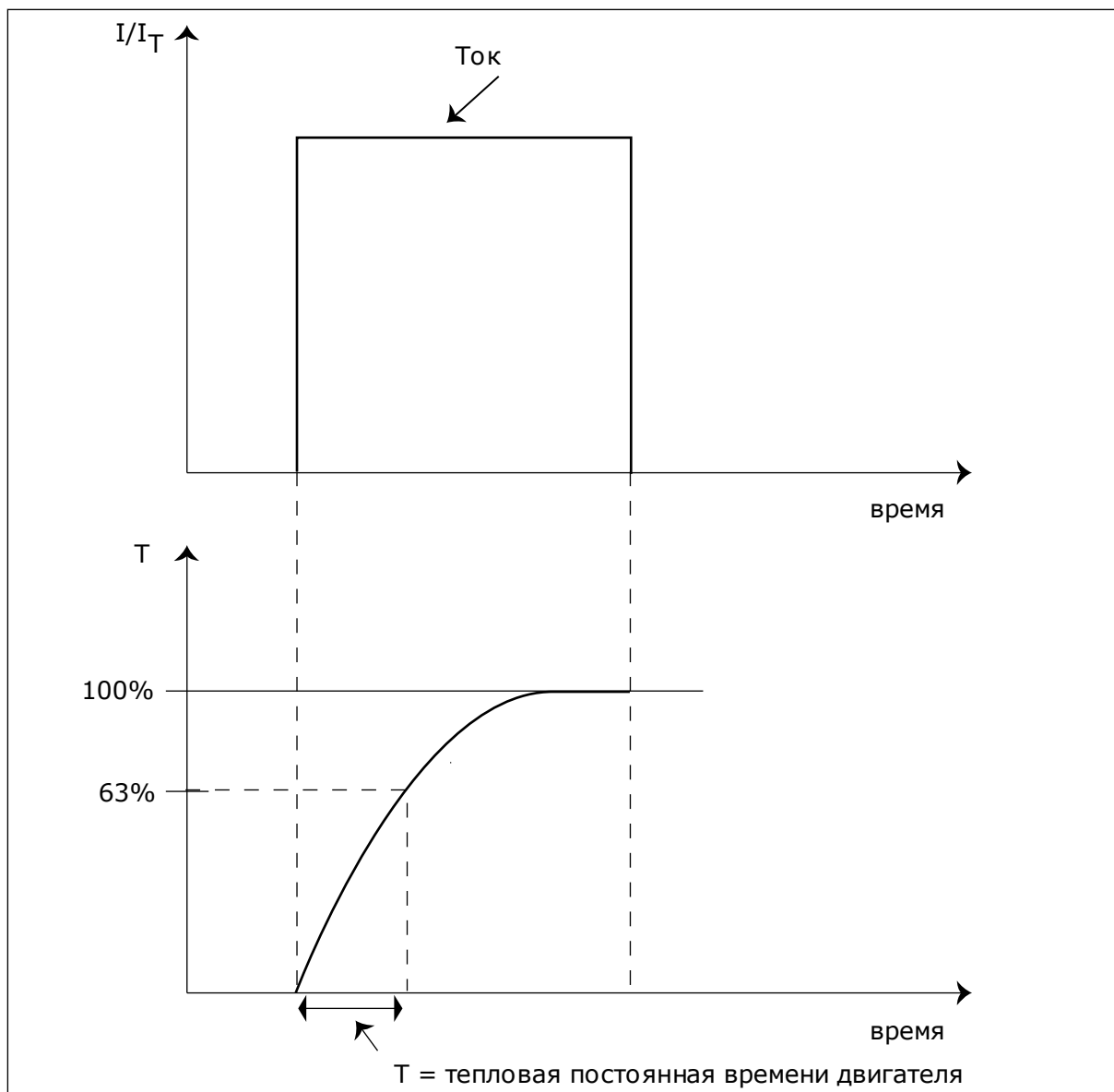
Рис. 65: Тепловая постоянная времени двигателя
