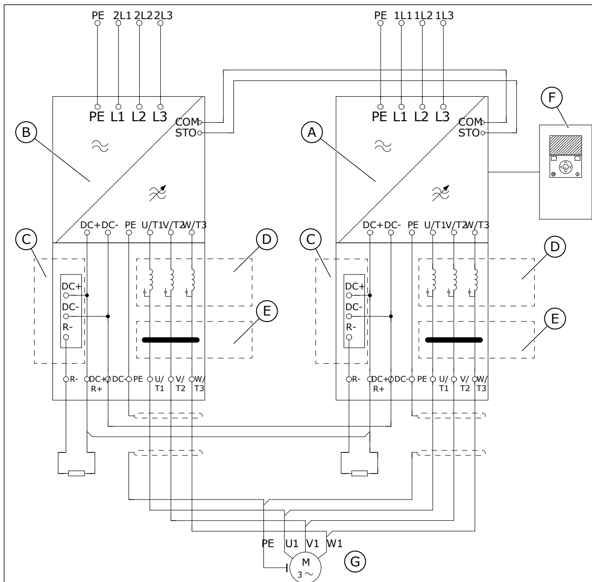
Рис. 12: Схема сети электроснабжения, MR12 с дополнительным модулем и дополнительными функциями
