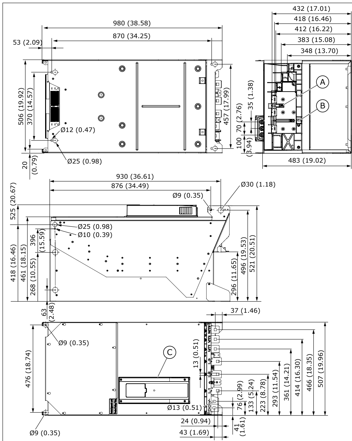
Рис. 5: Габариты без дополнительного модуля [мм (дюймы)]
