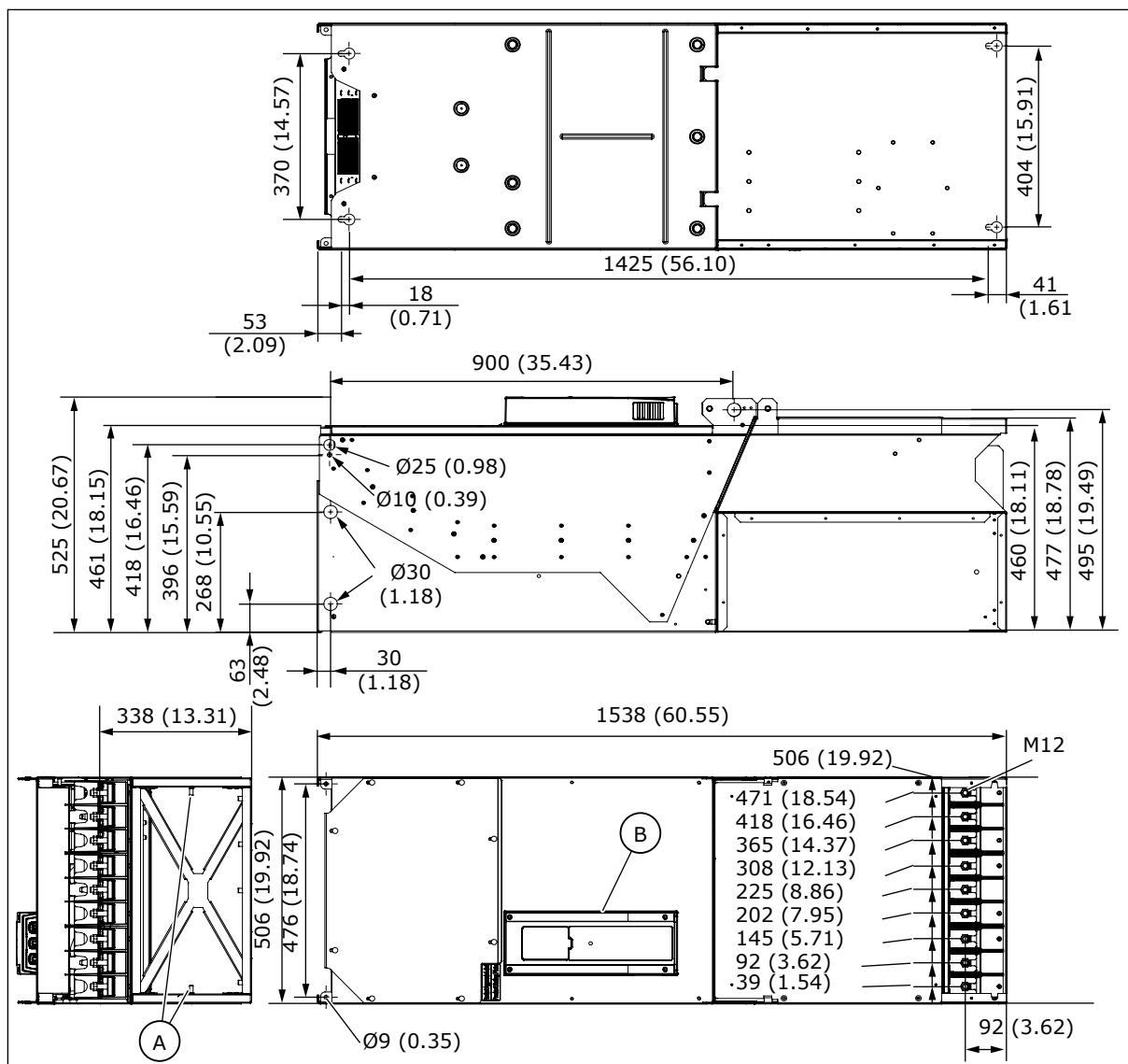
Рис. 7: Габариты с дополнительным модулем [мм (дюймы)]
