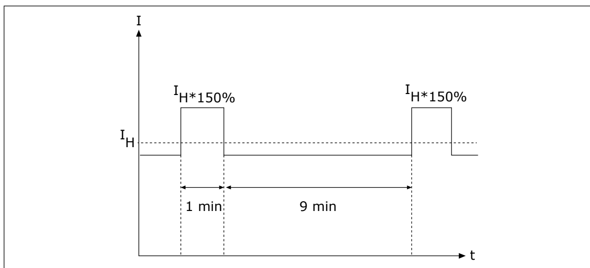
Рис. 27: Большая перегрузка
