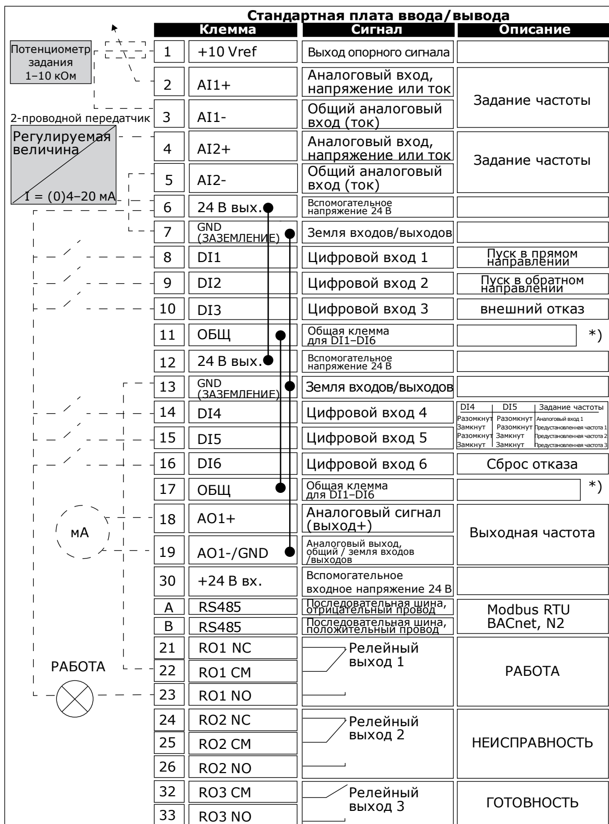
Рис. 19: Сигналы клемм управления привода на стандартной плате ввода/вывода и пример подключения. При заказе с дополнительным кодом +SBF4 релейный выход 3 замещается входом термистора.
