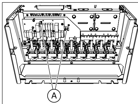
A. Электромагнитные перемычки
