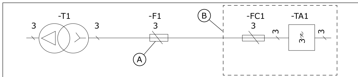
Рис. 16: Расположение предохранителей
