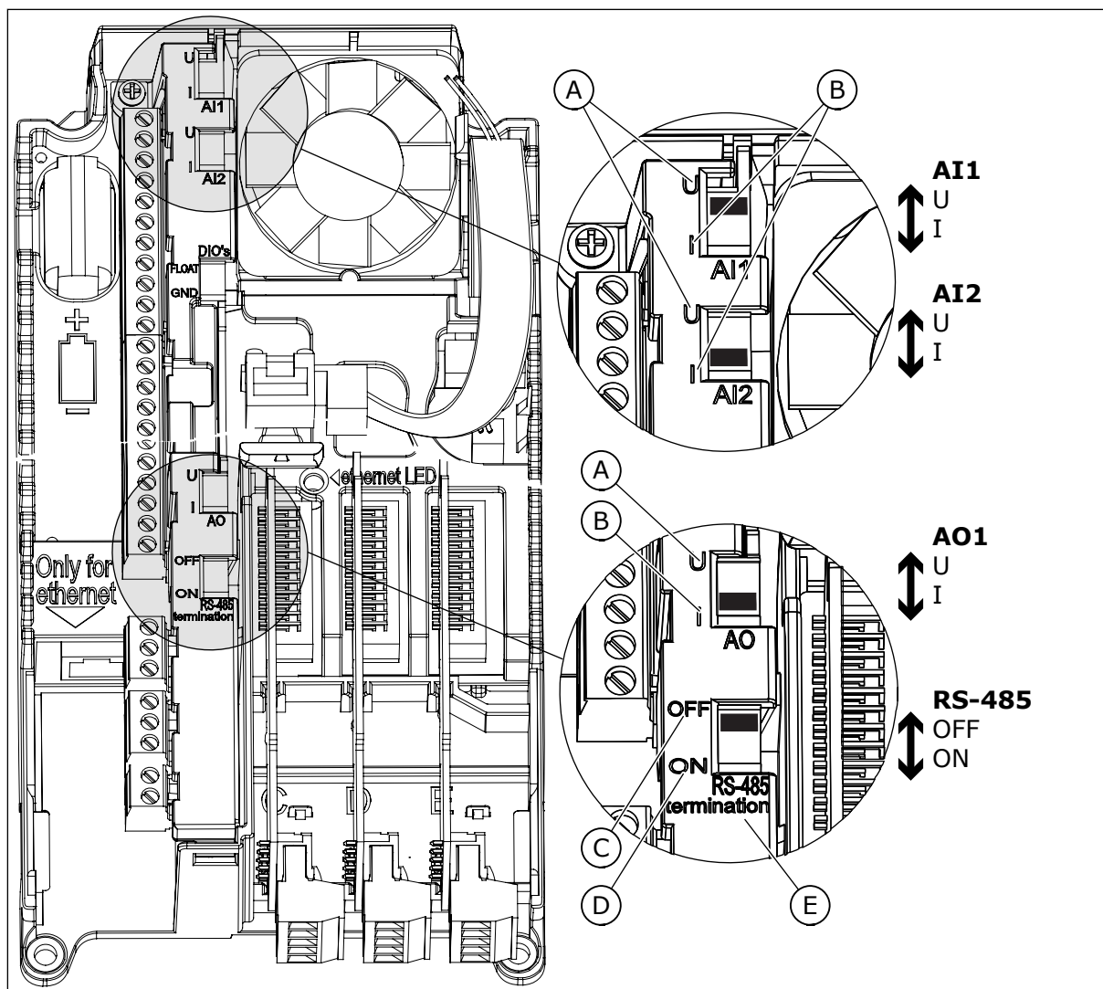
Рис. 22: Положения DIP-переключателей
