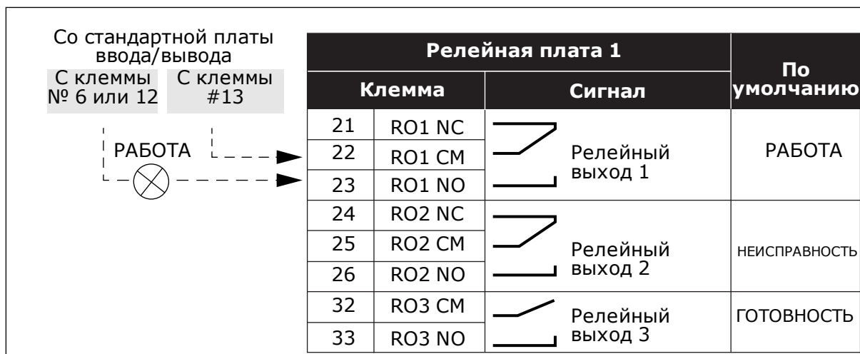
Рис. 20: Стандартная релейная плата (+SBF3)
