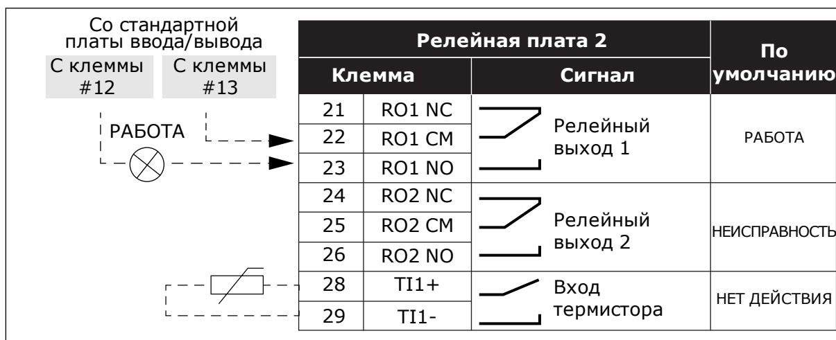
Рис. 21: Дополнительная релейная плата (+SBF4)
