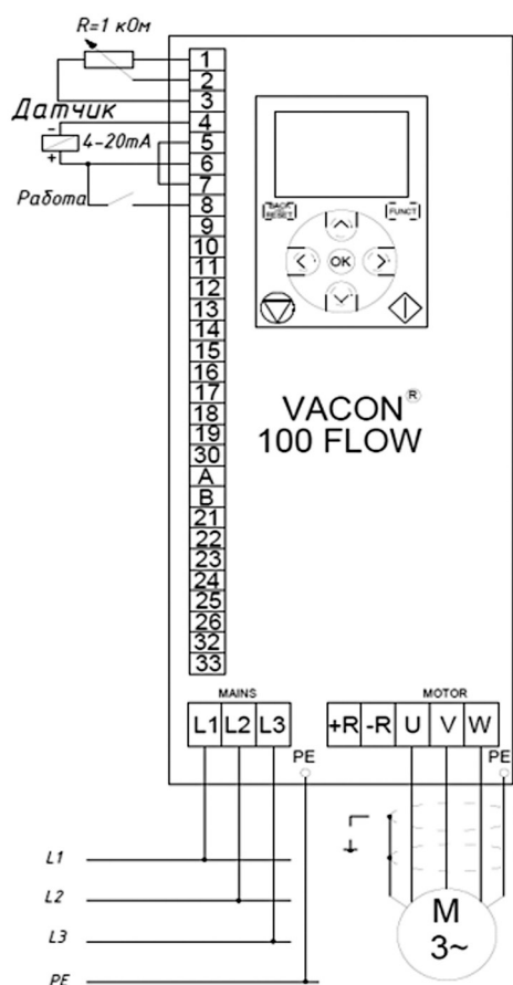
Рисунок 6. Режим поддержания постоянного давления, установка от потенциометра.
