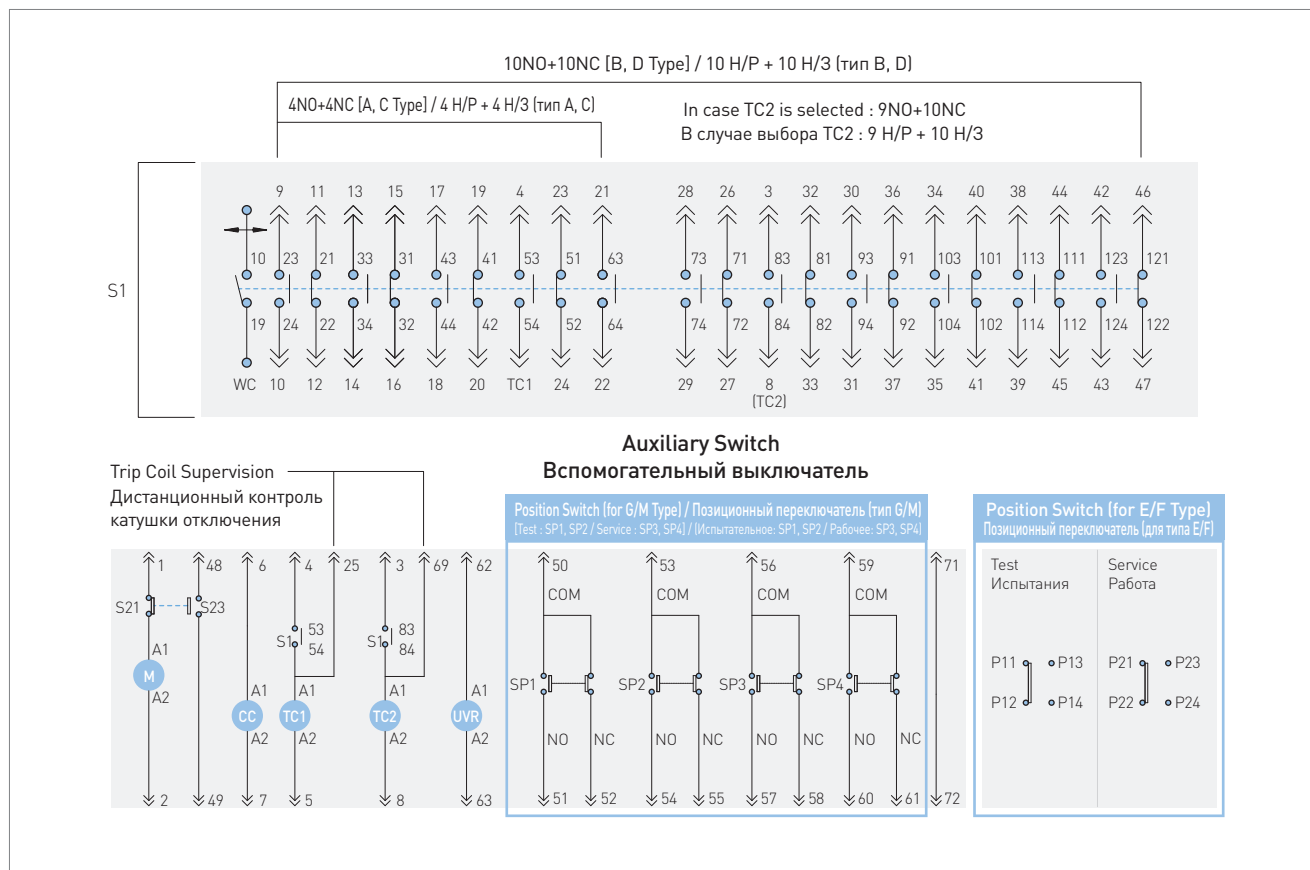
Fig. 2-2 Circuit diagram / Рис. 2-2 Электрическая схема
