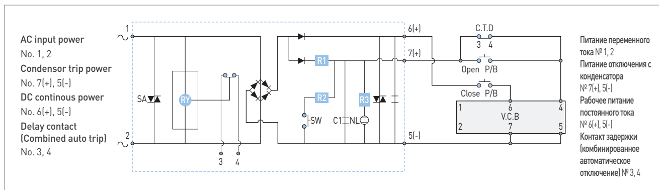
Fig. 2-6 Circuit diagram of condenser trip device / Рис. 2-6 Электрическая схема блока отключения конденсатора
