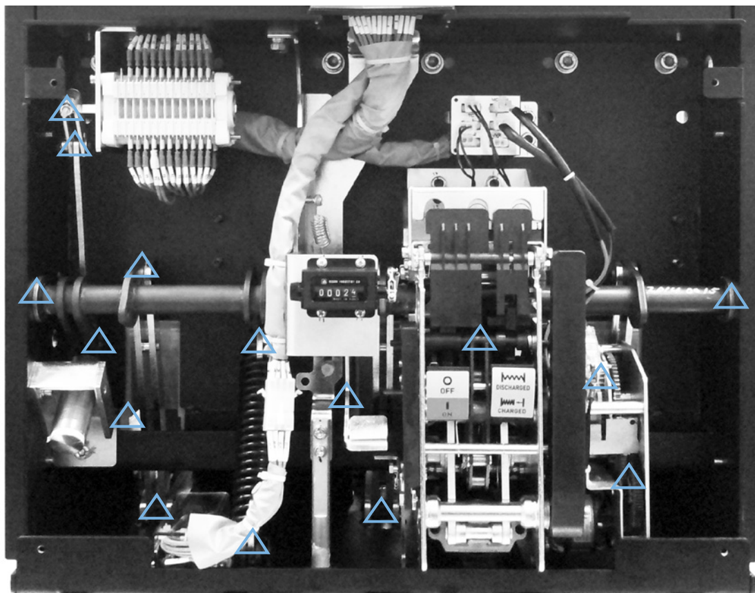
Fig. 5-2 Lubrication points / Рис. 5-2 Точки смазки
