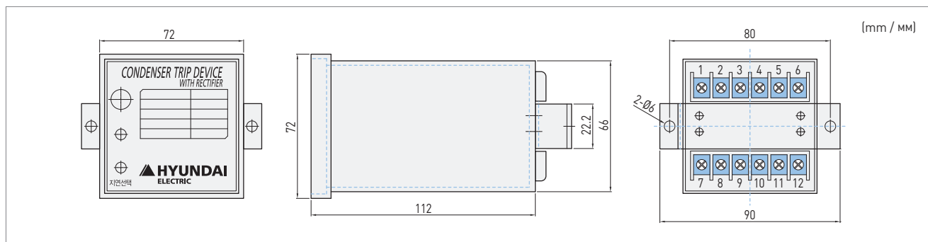
Fig. 2-5 Condenser trip device / Рис. 2-5 Блок отключения конденсатора
