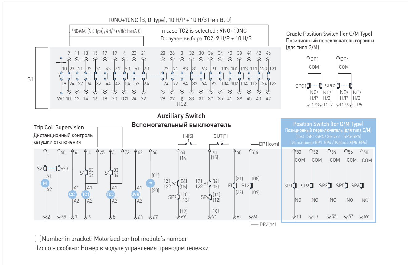
Fig. 2-3 Circuit diagram / Рис. 2-3 Принципиальная электрическая схема
