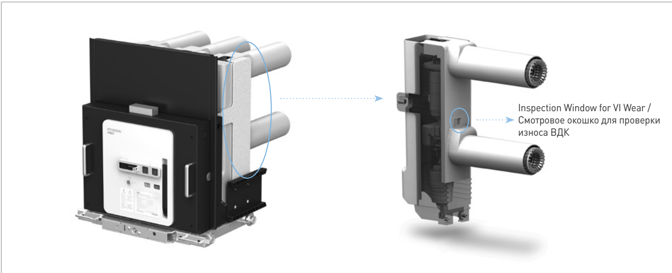
Fig. 5-1 Structure of the insulation frame / Рис. 5-1 Конструкция изоляционной рамы
