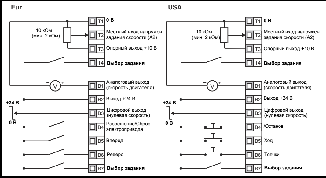
Рис. 10-27 Pr 11.27 = AV.Pr
