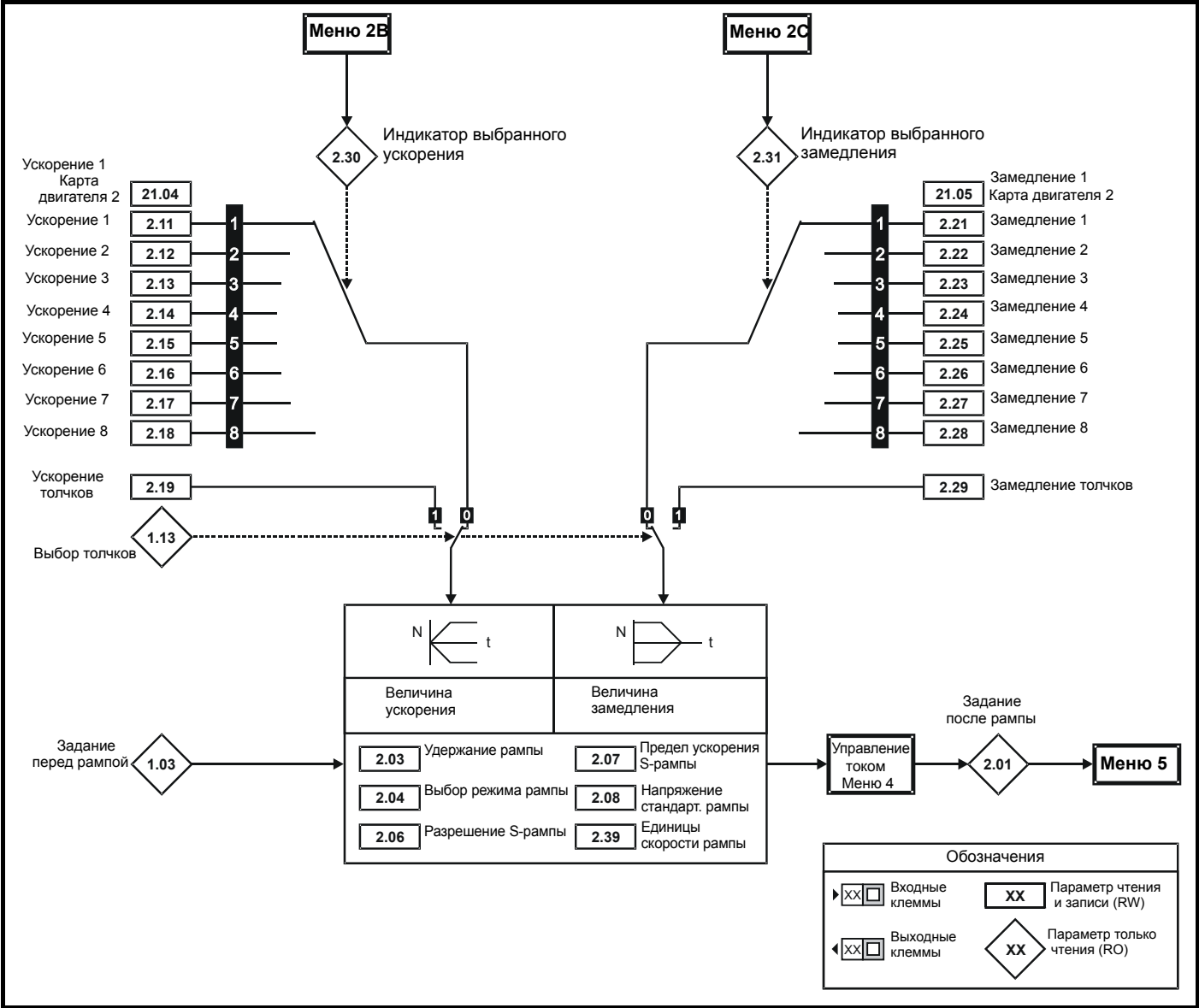
Рис. 10-5 Логическая схема меню 2A
