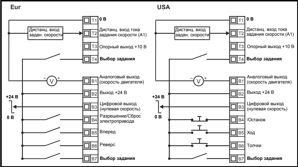
Рис. 10-28 Pr 11.27 = AI.Pr
