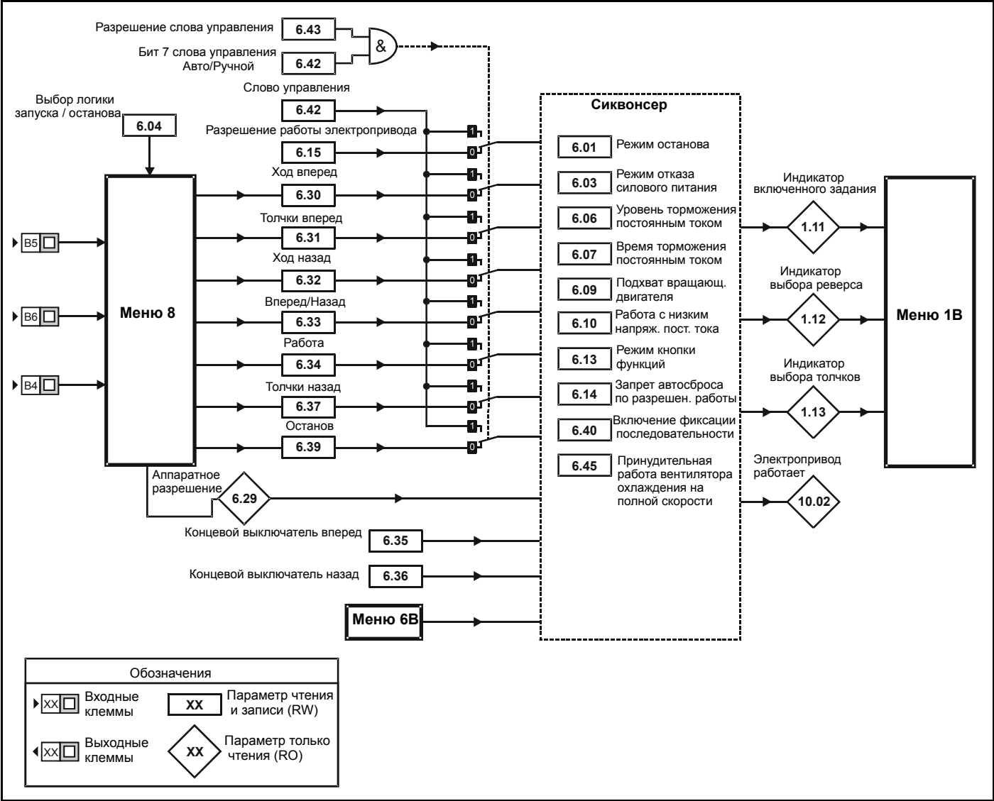
Рис. 10-14 Логическая схема меню 6А
