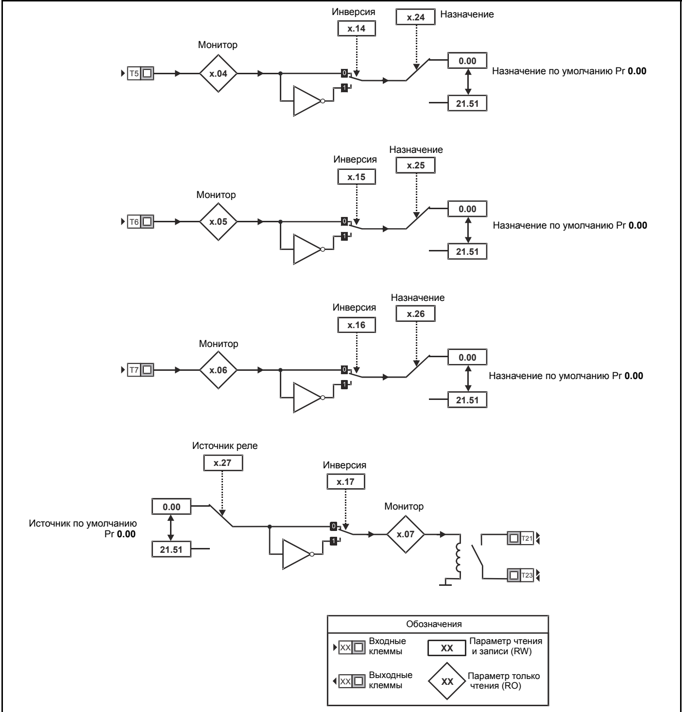
Рис. 10-44 Логическая схема меню 15А*
