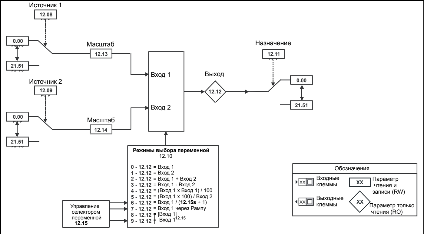
Рис. 10-38 Логическая схема меню 12С
