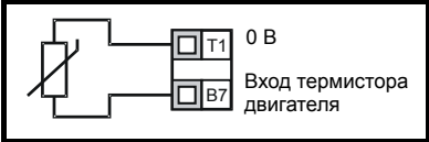
Рис. 10-22 Схема подключения термистора
