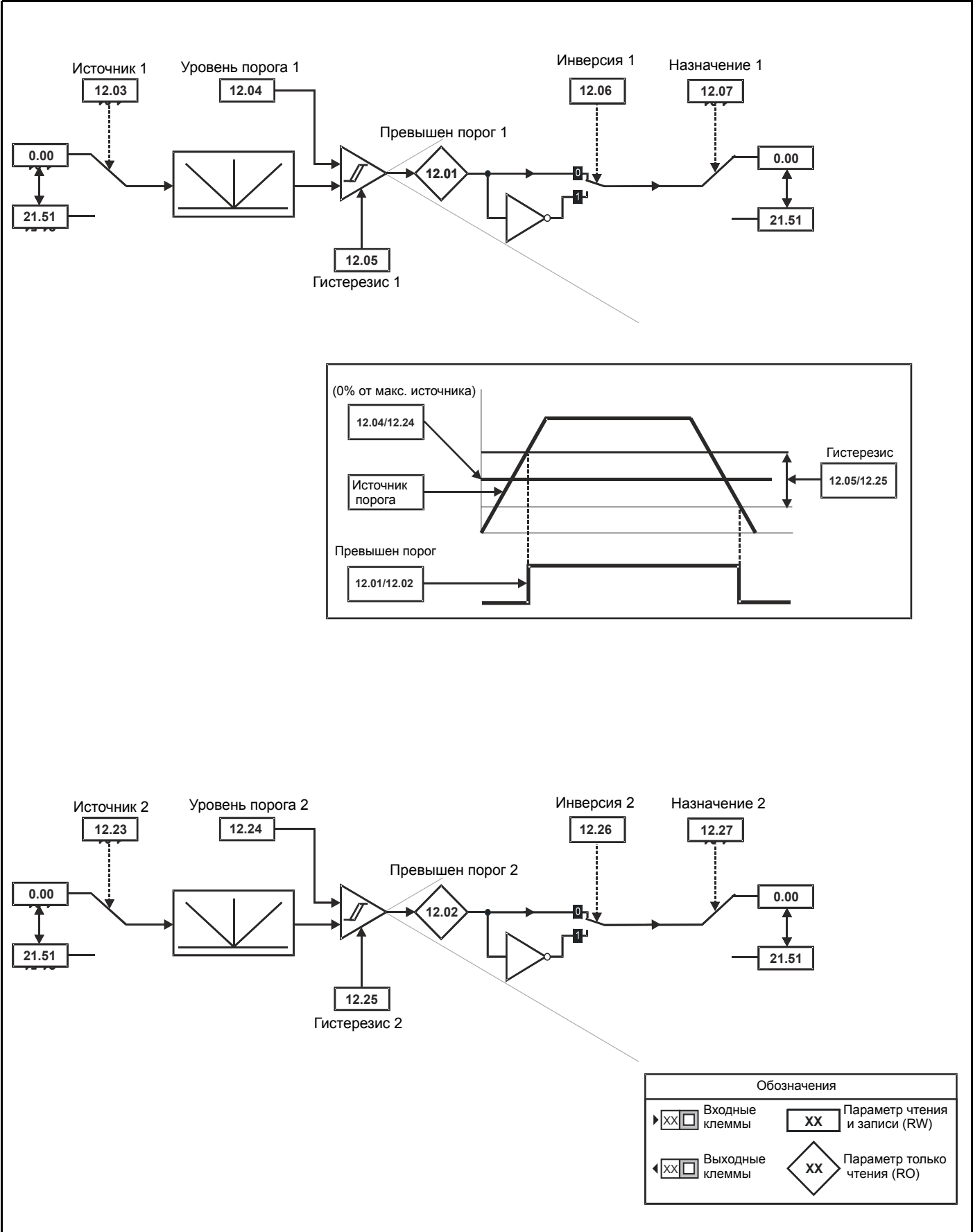
Рис. 10-36 Логическая схема меню 12A
