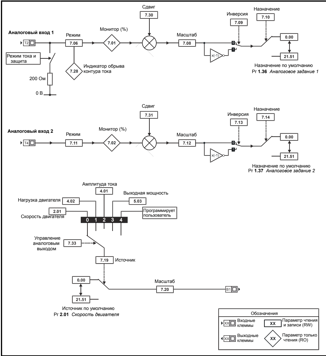
Рис. 10-17 Логическая схема Меню 7
