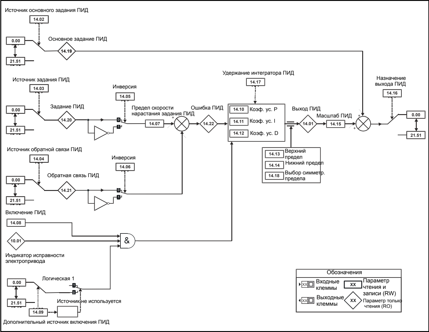
Рис. 10-42 Логическая схема Меню 14
