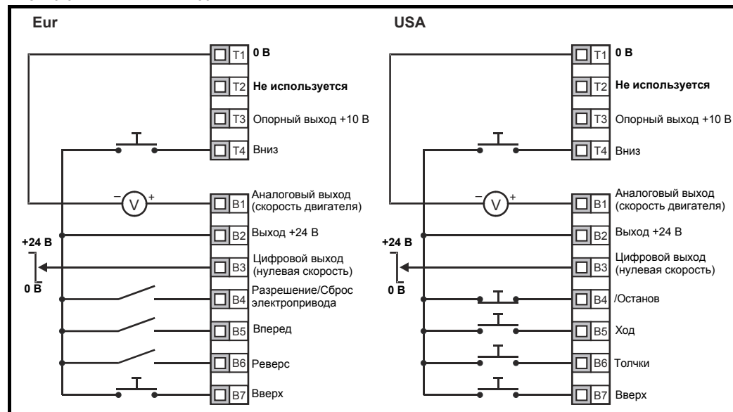
Рис. 10-31 Pr 11.27 = E.Pot
