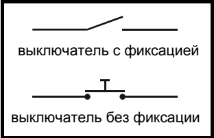
Рис. 10-25 Обозначения выключателей
