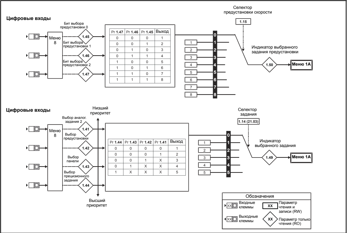
Рис. 10-3 Логическая схема меню 1С
