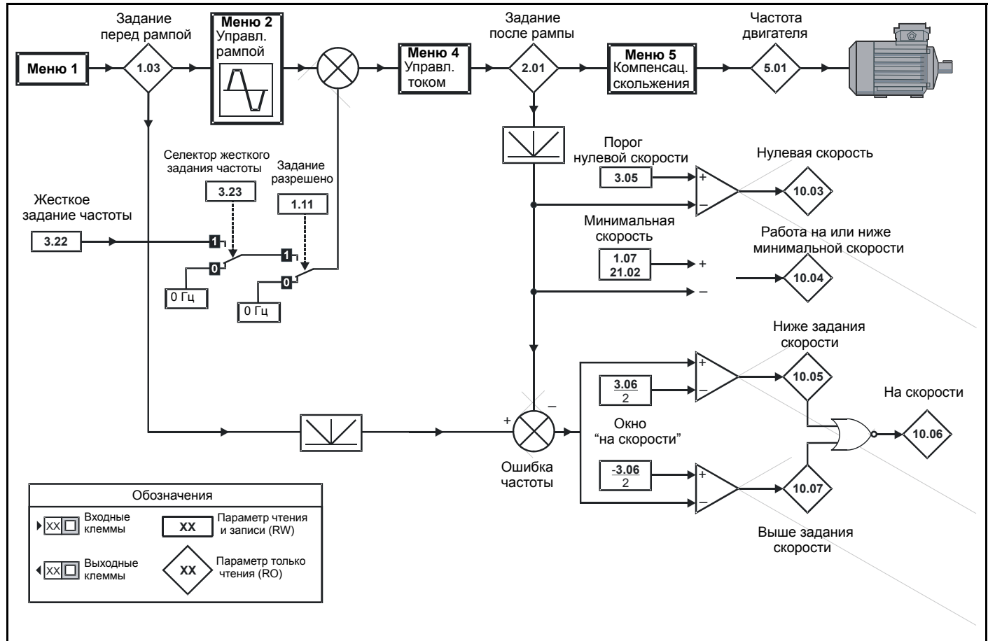
Рис. 10-10 Логическая схема меню 3А
