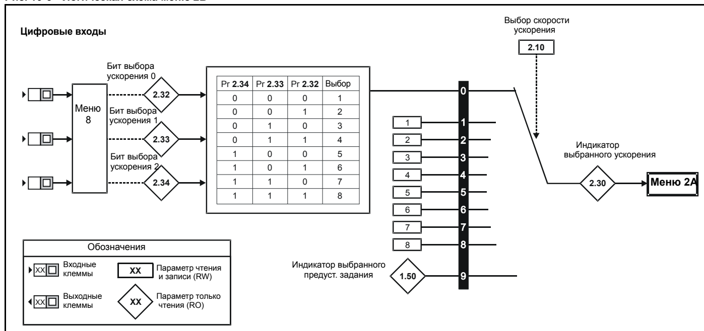
Рис. 10-7 Логическая схема меню 2С
