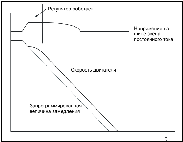
Рис. 10-8
