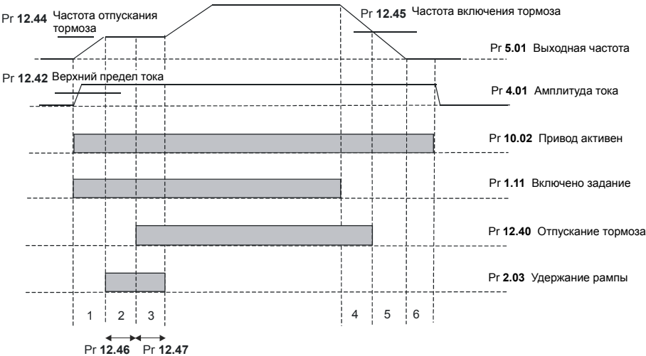
Рис. 10-41 Последовательность торможения
