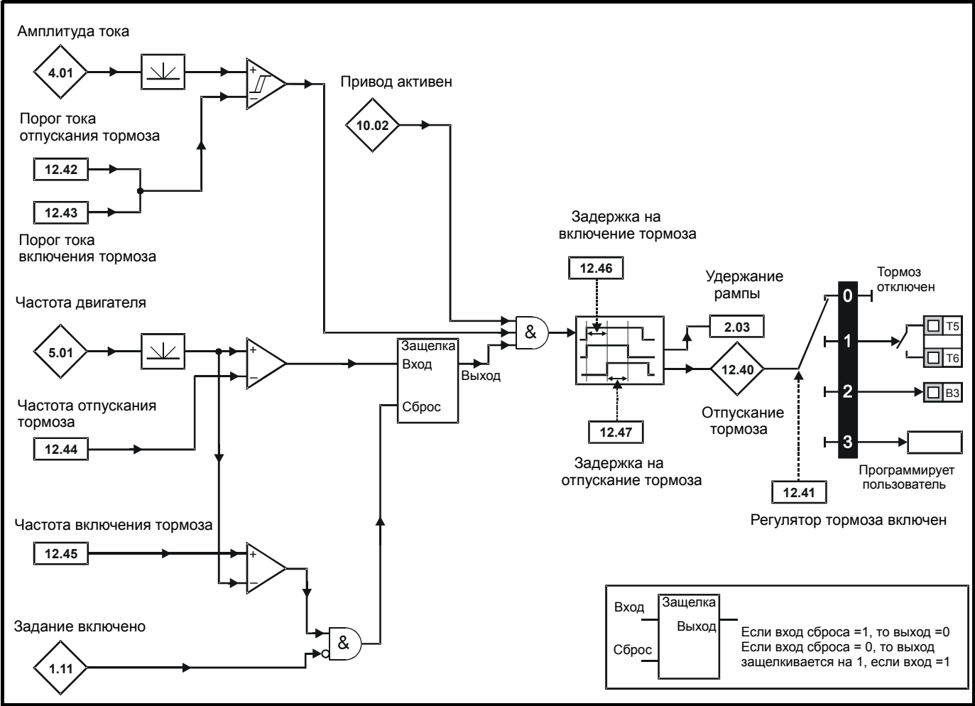
Рис. 10-41 Последовательность торможения
