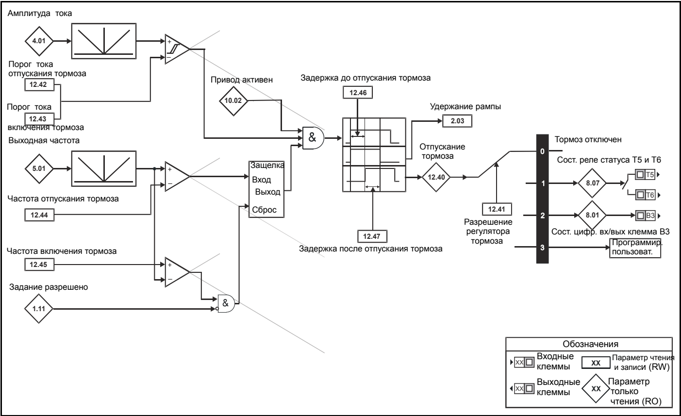
Рис. 10-39 Логическая схема меню 12D
