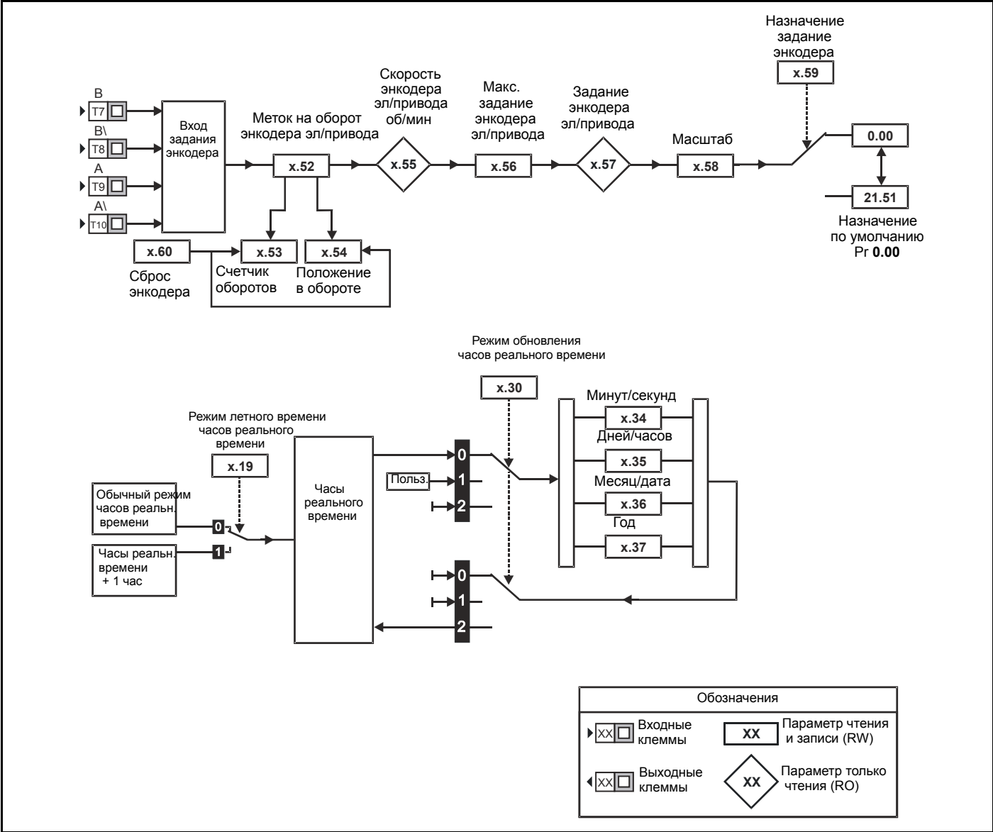
Рис. 10-46 Логическая схема меню 15C*
