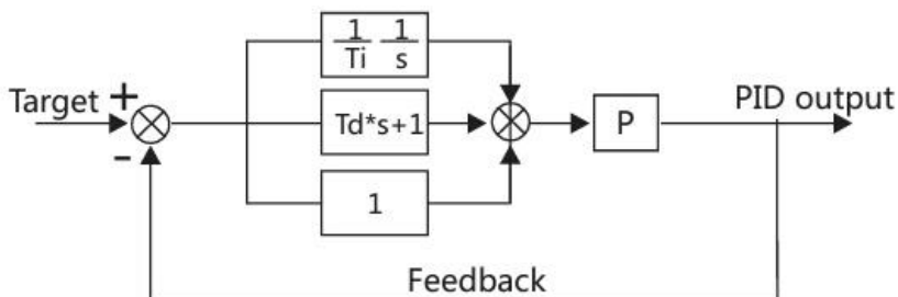
Рисунок 6-34 Принципиальная блок-схема ПИД-регулирования (Target – целевой сигнал, Feedback – обратная связь, PID output – выходной сигнал ПИД-регулятора)
