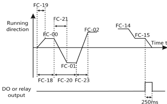
Рис. 6-39 Простой ПЛК в качестве источника частоты (Running direction – направление вращения, DO or relay output – цифровой или релейный выход, Time – время)
