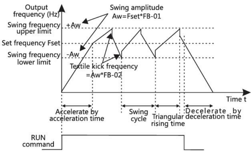
Рис. 6-37 Управление частотой качаний
