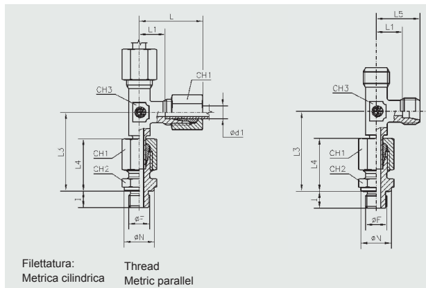
Forma B DIN 3852 Foglio 2
