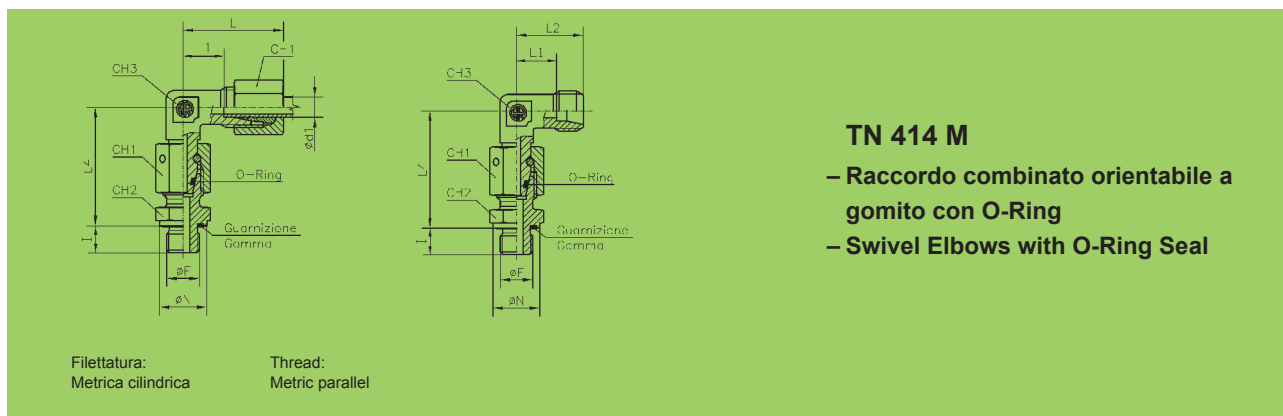
Forma E DIN 3852 Foglio 11
