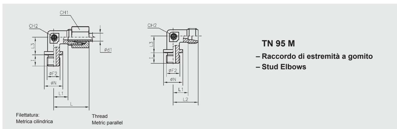
Forma B DIN 3852 Foglio 2 Type B DIN 3852 Part 2
