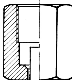
– Dado di serraggio – Tightening nut
