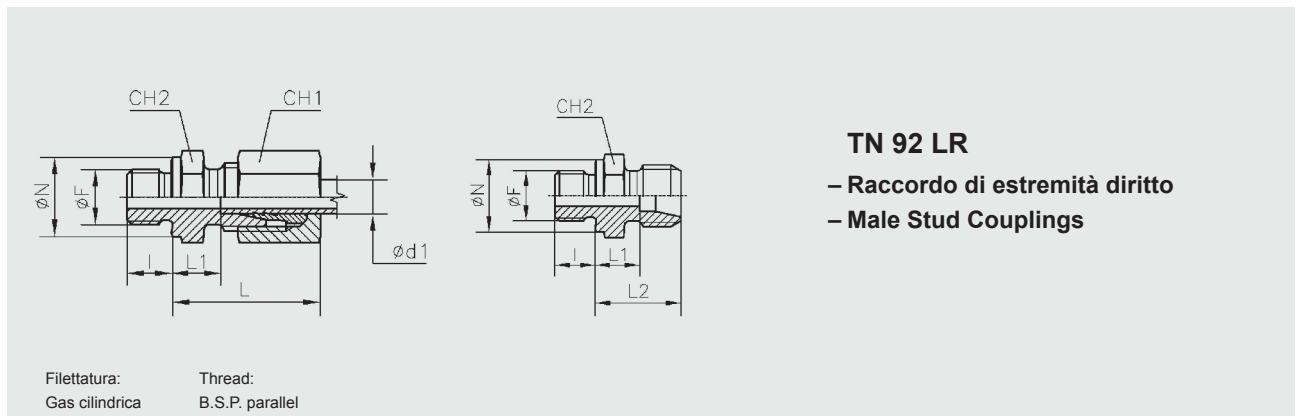
Forma B DIN 3852 Foglio 2
