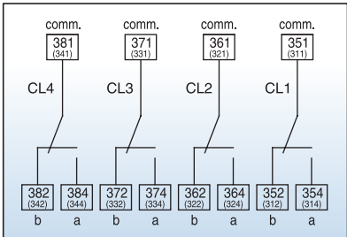
Блок контактов 4С с правой стороны корзины
