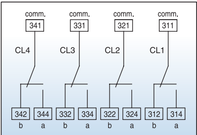
Блок контактов 4С с левой стороны корзины
