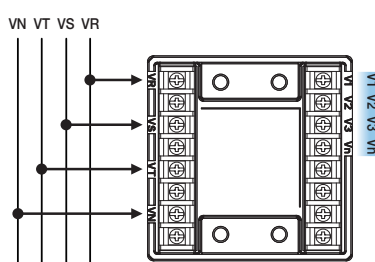
схема 3P4W (3 полюса, 4 обмотки)
