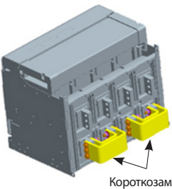
Короткозамыкающая шина
