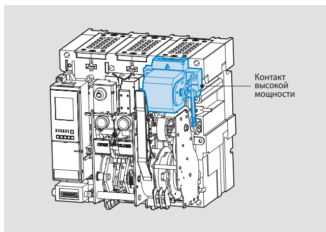
Тип вспом. контакта и взвода пружины
