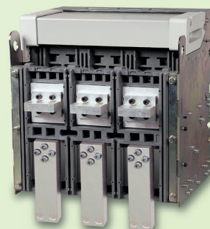
Горизонтальные выводы/выводы для подключения шин спереди
