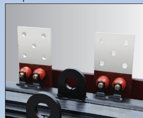
Клеммы заземления
