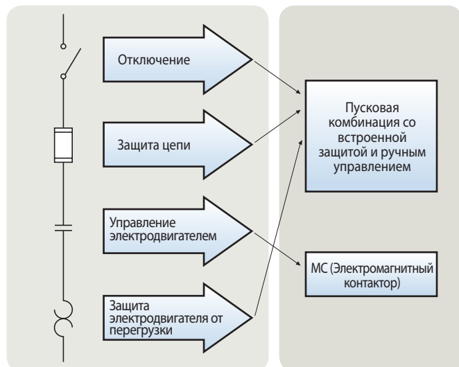
Функции управления электродвигателем
