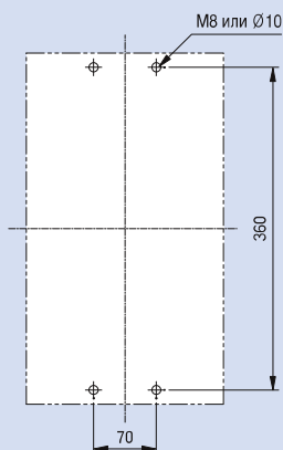
Разметка отверстий в монтажной панели
