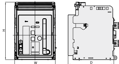
Выкатной тип
