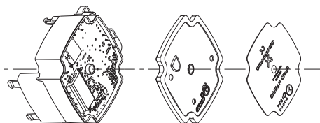
Рис. 50 Блок управления
