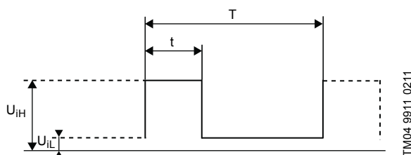
Рис. 12 ШИМ-сигнал
