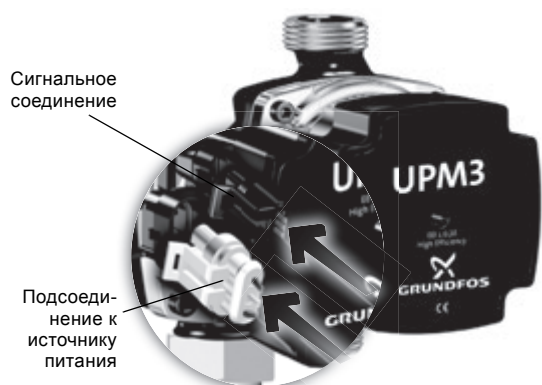
Рис. 61 Подключение кабеля питания и сигнальное соединение.
