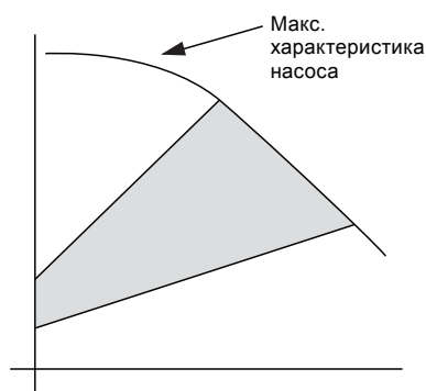
Рис. 30 Рабочая область функции AUTO_{ADAPT} для пропорционального давления
