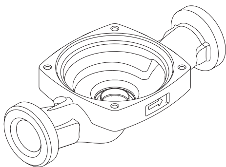
Рис. 49 Корпус насоса
