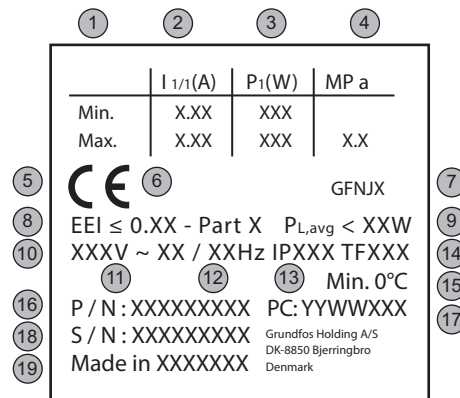
Рис. 8 Сторона клеммной коробки
