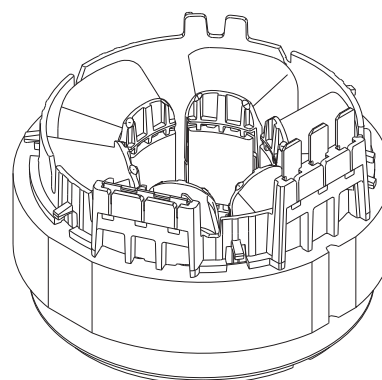
Рис. 38 Статор
