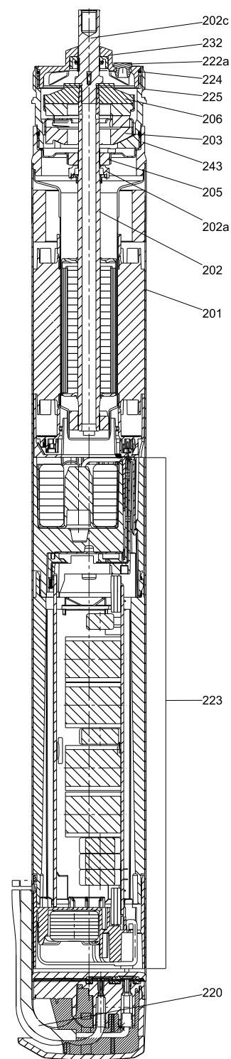
Рис. 31 MSF 3
