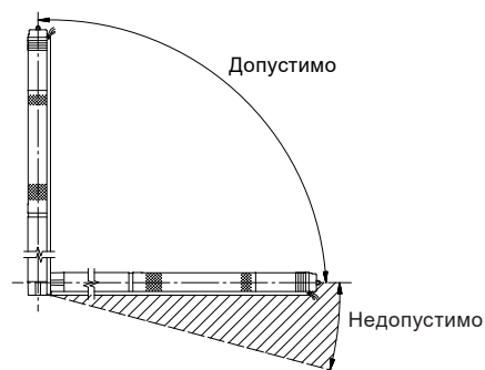
Рис. 4 Монтаж насосов SQF
