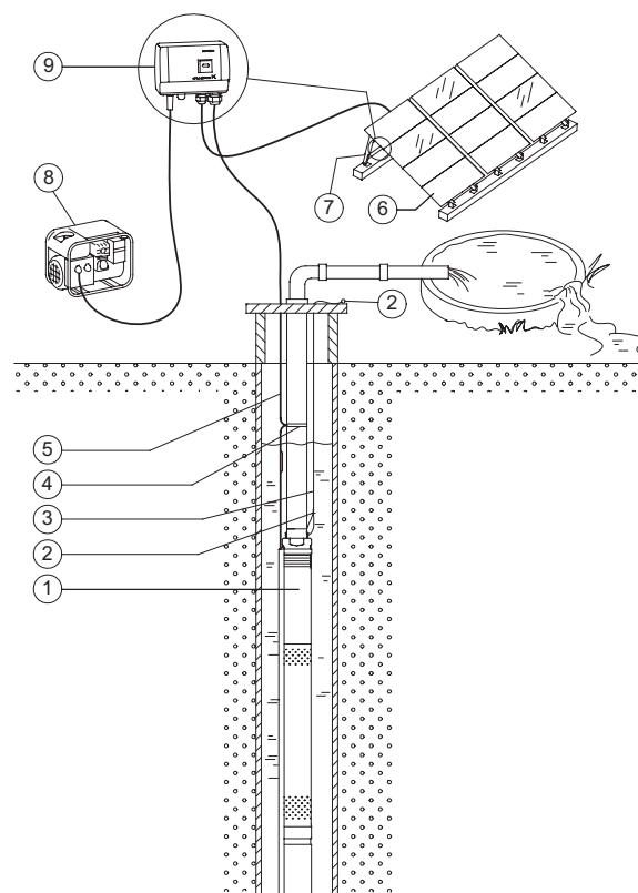
Рис. 8 Система SQFlex Solar с резервным генератором
