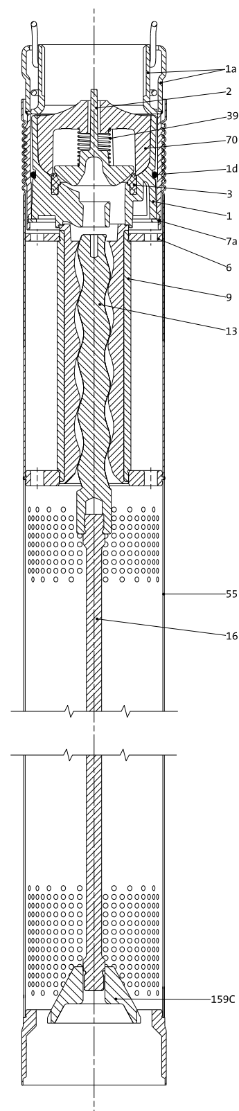
Рис. 27 пример: SQF 1.2-2
