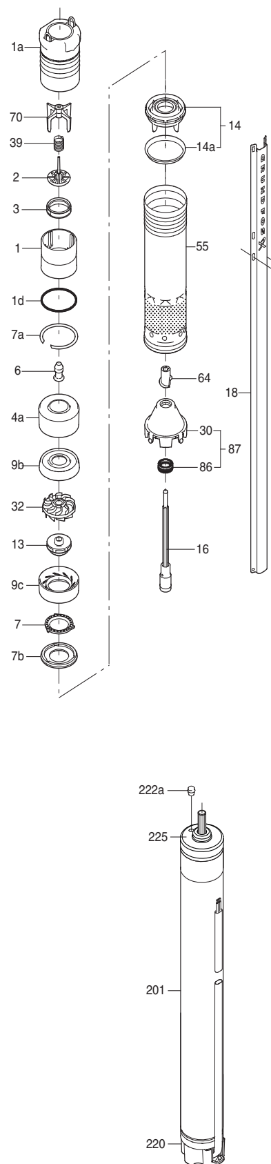
Рис. 28 Пример SQF 1-30
