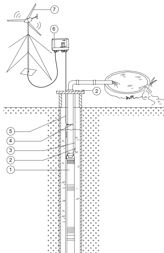
Рис. 11 SQFlex Wind
