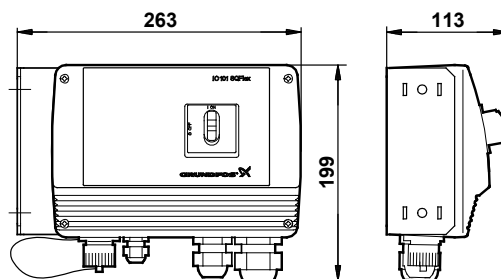
Рис. 23 Размеры, IO 101
