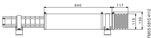
Рис. 34 Кожух охлаждения и сетчатый фильтр для SQF 4"
