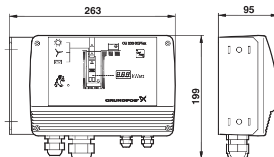
Рис. 19 Размеры, CU 200
