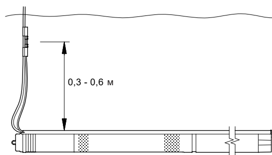
Рис. 5 Горизонтальный монтаж
