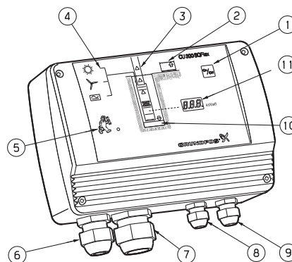
Рис. 18 Компоненты блока CU 200
