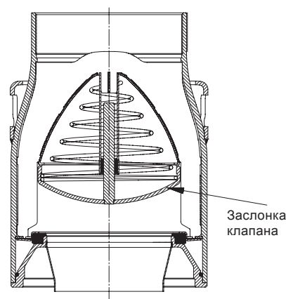
Рис. 5 Обратный клапан
