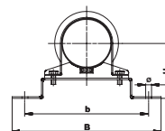
Накладной хомут
