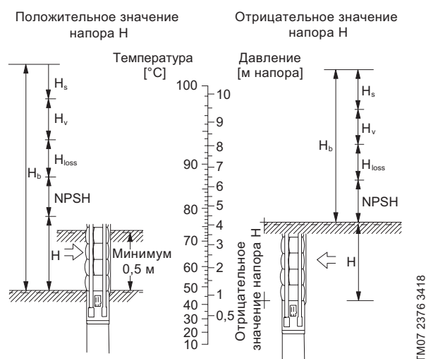
Рис. 20 Глубина установки
