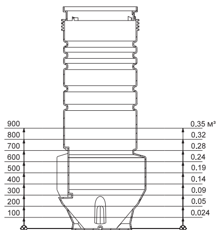
Рис. 140 Полезный объем относительно уровня, PS.R.08
