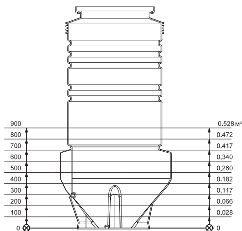
Рис. 142 Полезный объем относительно уровня, PS.R.10
