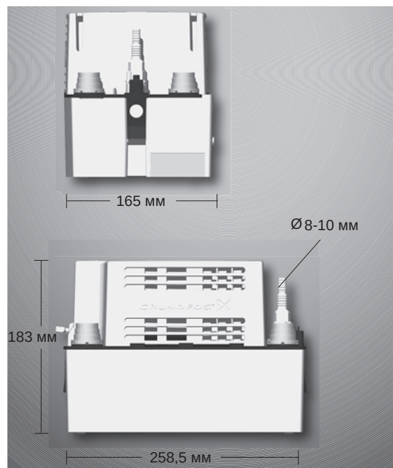
Рис. 74 Габаритные размеры
