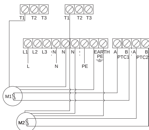
Рис. 117 Однофазные подключения для двух насосов
