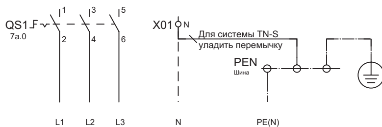
Сеть электропитания
