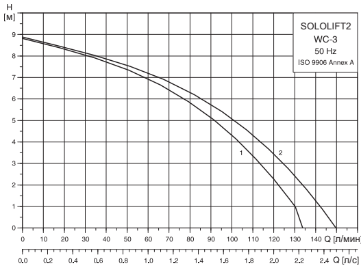
Рис. 59 Кривые характеристик
