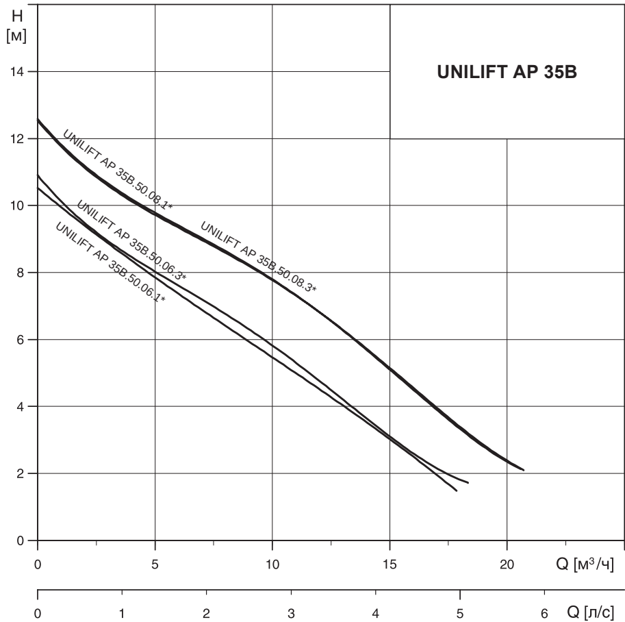
Рис. 28 Кривые характеристик
