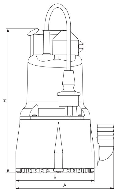
Рис. 39 Размеры KPC 24/7
