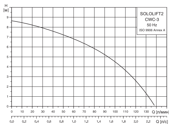
Рис. 62 Кривые характеристик
