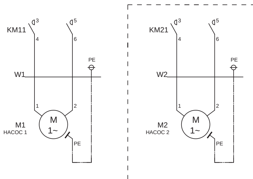
Рис. 122 Подключение однофазных насосов с конденсаторами
