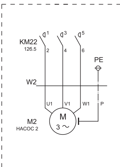
Рис. 125 Подключение трехфазных насосов по схеме прямого включения (DOL)
