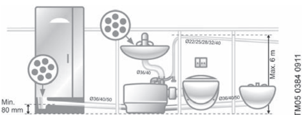
Рис. 50 Для подвесного унитаза, раковины, душевой кабины и биде (SOLOLIFT2 CWC-3)
