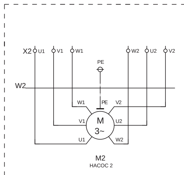
Рис. 126 Подключение трехфазных насосов по схеме "звезда-треугольник" (SD)
