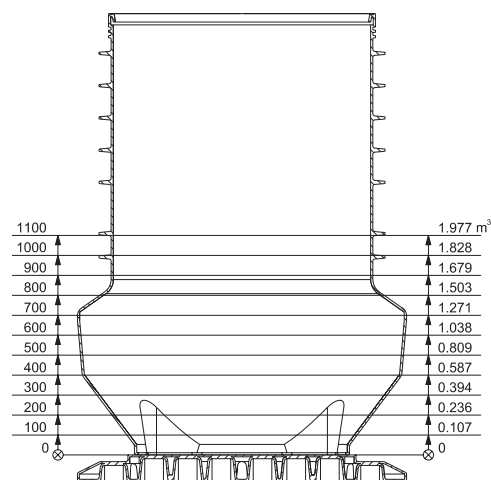
Рис. 144 Полезный объем относительно уровня, PS.R.17
