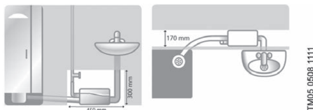
Рис. 52 Для раковины и душевой кабины (SOLOLIFT2 D-2)
