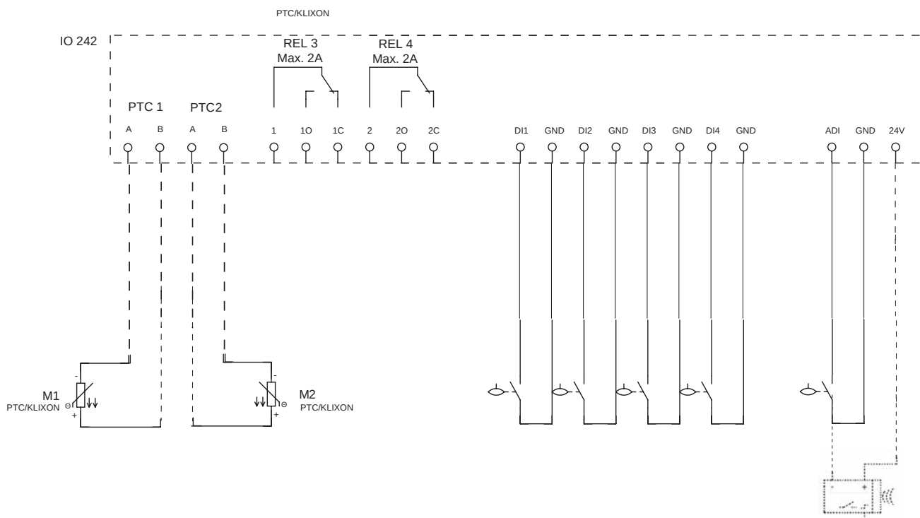
Рис. 130 Подключение сигнальных цепей. Шкаф управления двумя насосами
