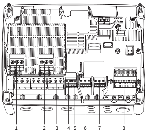
Рис. 118 Клеммные колодки
