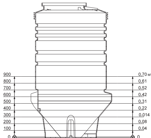
Рис. 143 Полезный объем относительно уровня, PS.R.12 (один насос)
