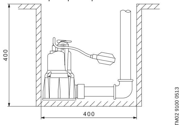
Рис. 34 Минимальные размеры приемка для насоса KPC 300 A
