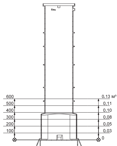
Рис. 139 Полезный объем относительно уровня, PS.R.05
