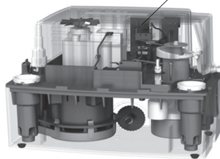
Рис. 73 Пример установки системы контроля Alarm PCB CONLIFT в насосе CONLIFT1
