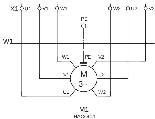
Рис. 126 Подключение трехфазных насосов по схеме "звезда-треугольник" (SD)
