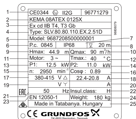
Рис. 4 Фирменная табличка
