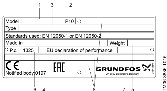
Рис. 4 Фирменная табличка насосных станций PS.G
