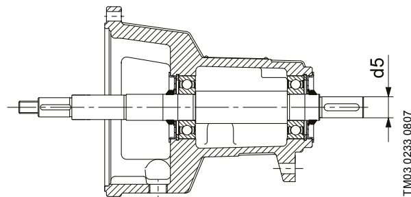
Рис. 23 Подшипниковый узел и вал
