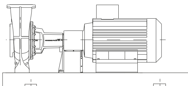
Рис. 85 Насос NKG с рамой-основанием EN/ISO
