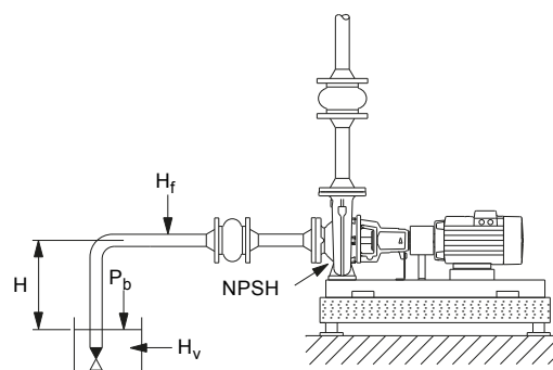
Рис. 41 Высота всасывания воды при положительном значении H_{всac}
