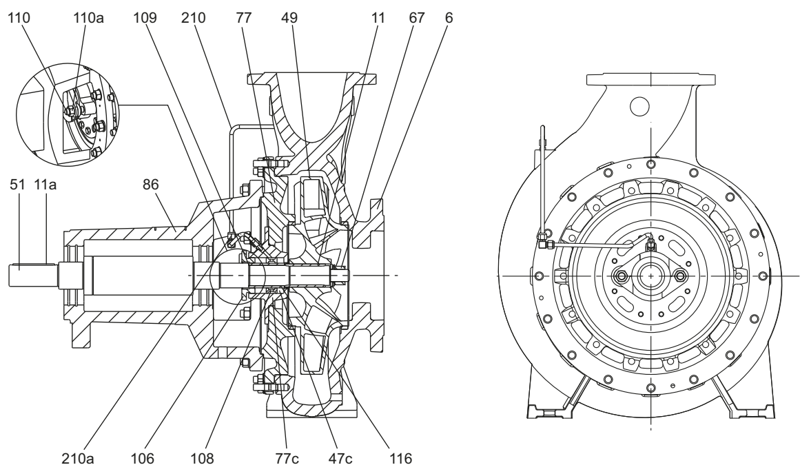
Рис. 11 Чертеж в разрезе, сальник с разъемной крышкой
