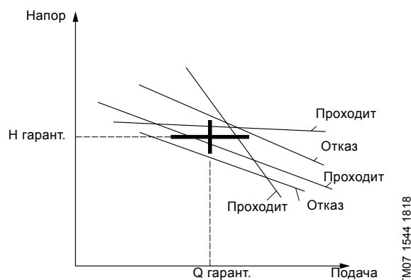
Рис. 68 Кривые насоса, которые проходят через допустимую область гарантируемой точки или не попадают в нее
