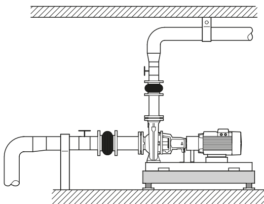
Рис. 50 Монтаж трубопровода
