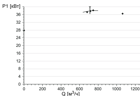
Рис. 72 Результаты измерения потребляемой мощности
