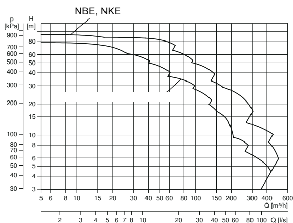
Рис. 55 Диапазон характеристик Е-насосов
