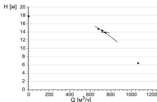
Рис. 69 Результаты измерения для подачи и напора
