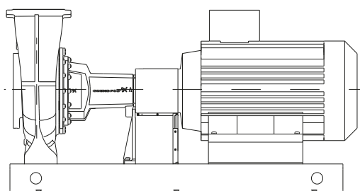
Рис. 79 Насос NK с С-образной рамой-основанием
