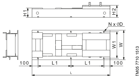
Рис. 85 С-образная рама-основание с 6 установочными отверстиями
