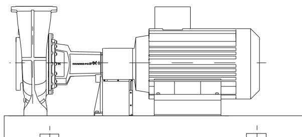
Рис. 78 Насос NK на раме-основании
