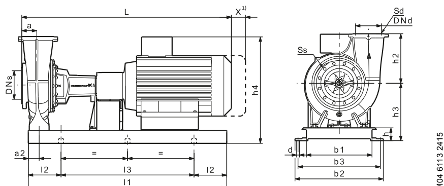
С-образная рама-основание, тангенциальный отвод
