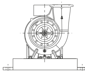
Рис. 26 Схематичное изображение насоса NK в сборе на раме-основании EN/ISO
