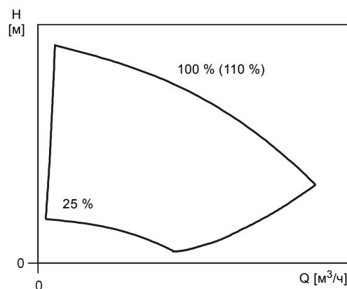
Рис. 56 Рабочий диапазон Е-насосов
