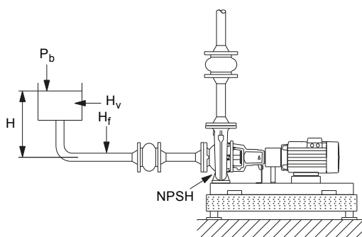
Рис. 42 Высота всасывания воды при отрицательном значении H_{всac}
