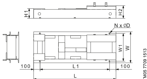
Рис. 84 С-образная рама-основание с 4 установочными отверстиями
