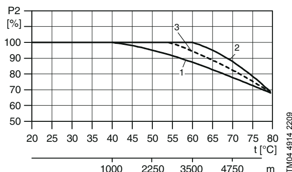
Рис. 32 Мощность двигателя в зависимости от температуры / высоты над уровнем моря
