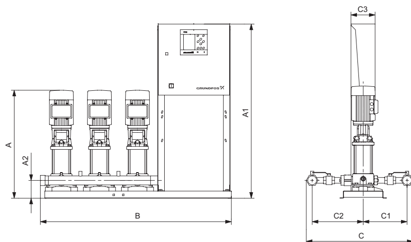
Рис. 54 Габаритный чертёж установки повышения давления Hydro MPC со шкафом управления, который смонтирован на одной раме-основании с насосами (исполнение A). Установка повышения давления приведена в качестве примера. Входящие в поставку насосы могут отличаться от показанных на схеме.
