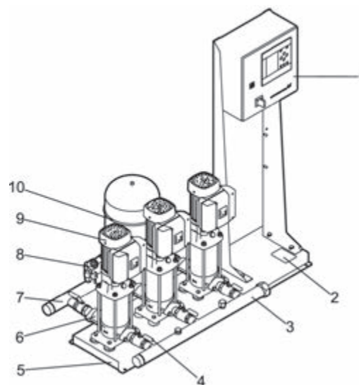
Рис. 8 Компоненты установки
