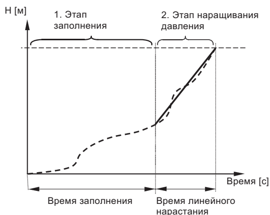
Рис. 98 Этапы заполнения и нарастания давления
