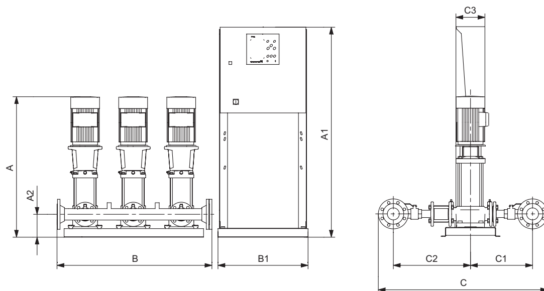
Рис. 64 Габаритный чертёж установки повышения давления Hydro MPC со шкафом управления, смонтированным на отдельной раме-основании (исполнение D). Установка повышения давления приведена в качестве примера. Входящие в поставку насосы могут отличаться от показанных на схеме.
