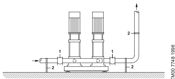
Рис. 121 Крепление трубопровода
