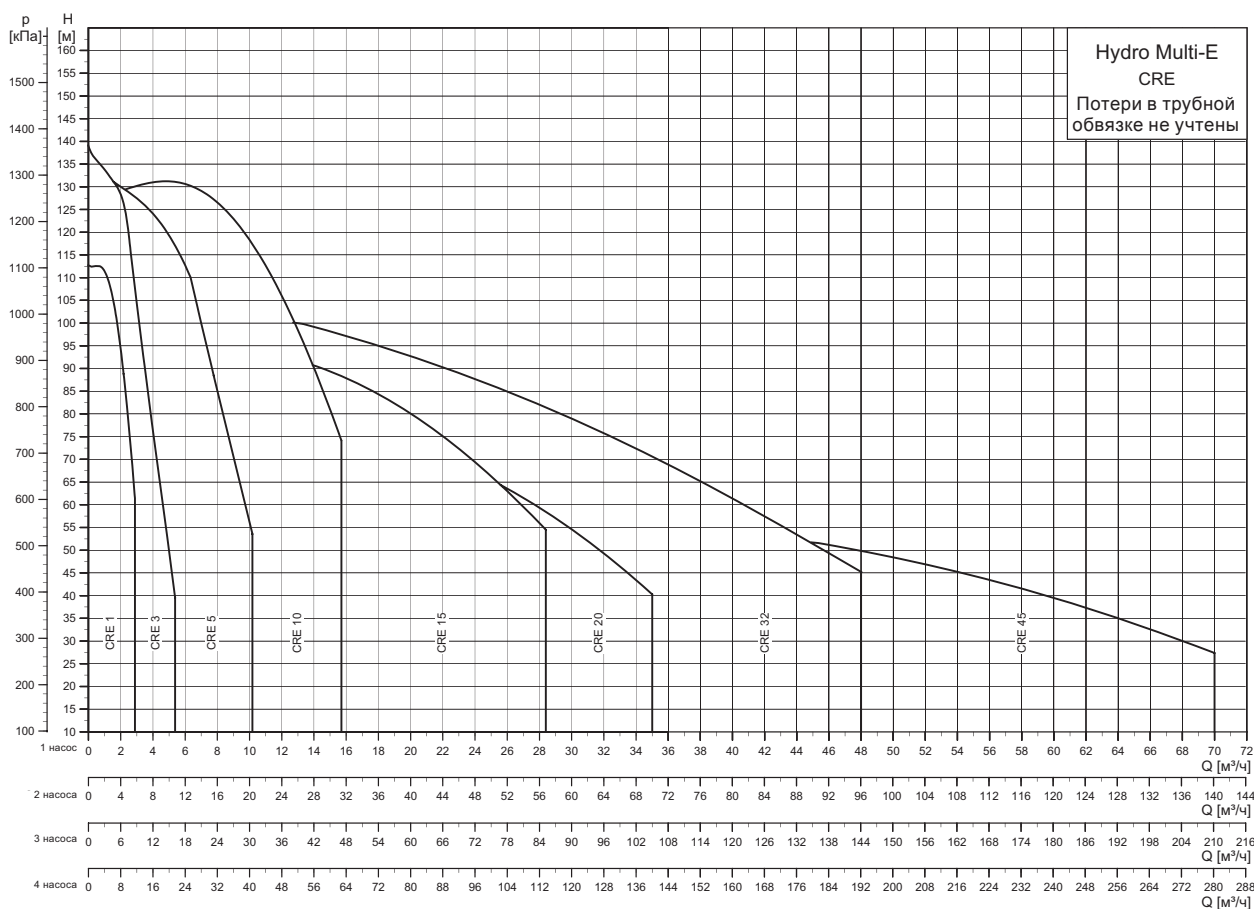
Рис. 91 Диапазон характеристик установок Hydro Multi-E с насосами CRE
