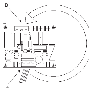
Рис. 119 Электронная печатная плата
