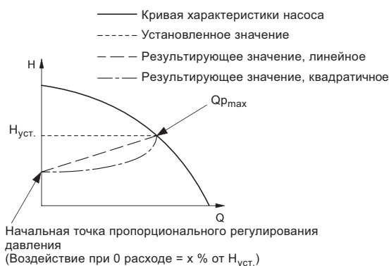
Рис. 28 Пропорциональное регулирование давления
