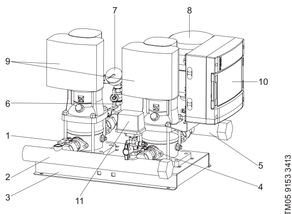
Рис. 94 Установка Hydro Multi-E с двумя насосами CRE
