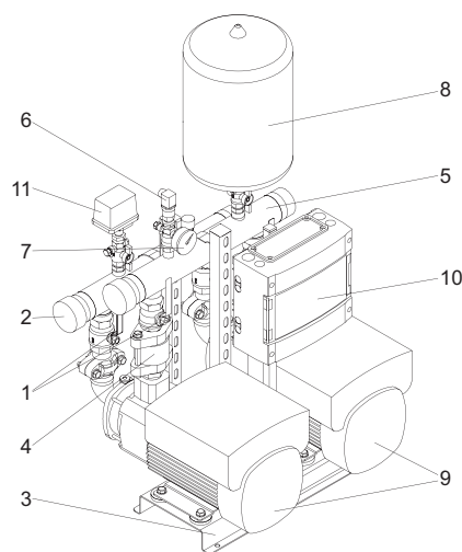
Рис. 95 Установка Hydro Multi-E с двумя насосами CME
