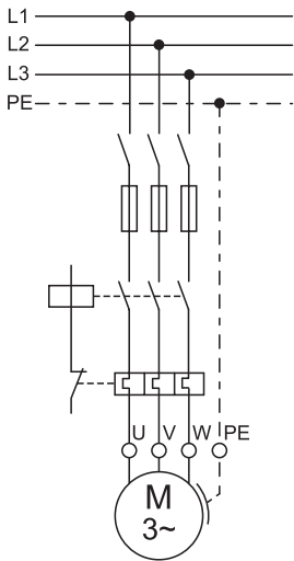
DOL
