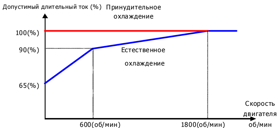
[Характеристика длительного тока для 4-х полюсного двигателя, 60 Гц]
