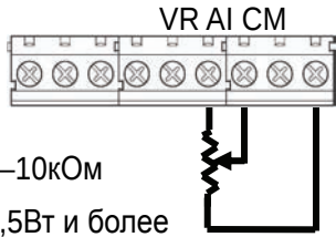
3) Исп. клеммы V.R
